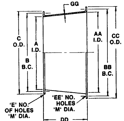
Inlet/Outlet Cone
